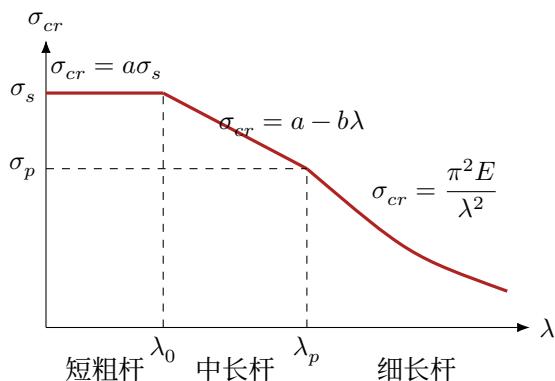
图 23: 临界应力总图
