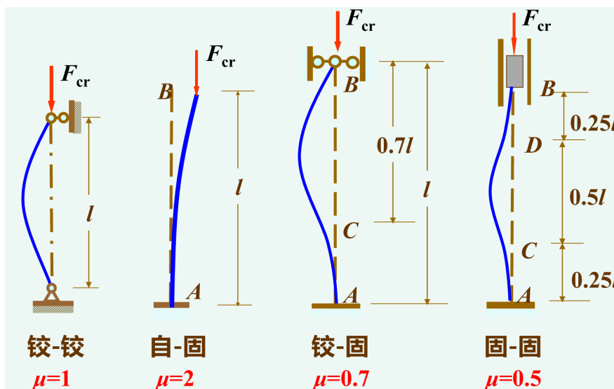
图 22: 不同端部约束下压杆屈曲形态示意
